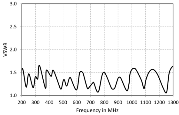
Fig. 1: VSWR (typ.)
